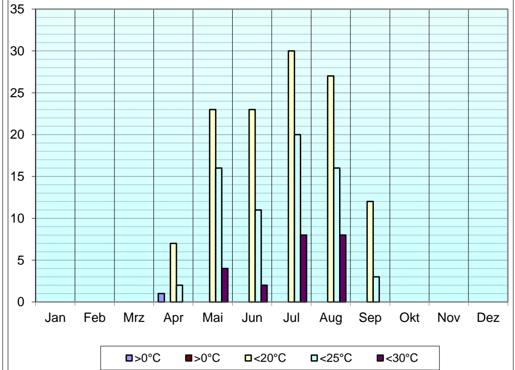
Temperatur Kenntage
