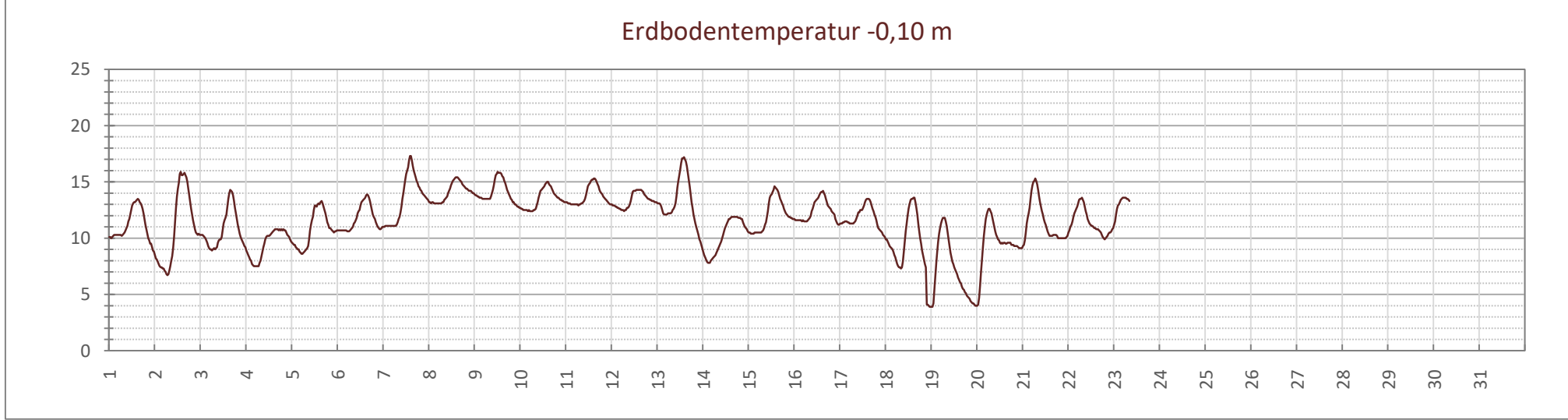
Diagramm der Erdbodentemperatur in 0,10 m tiefe im 10-Min-Takt
