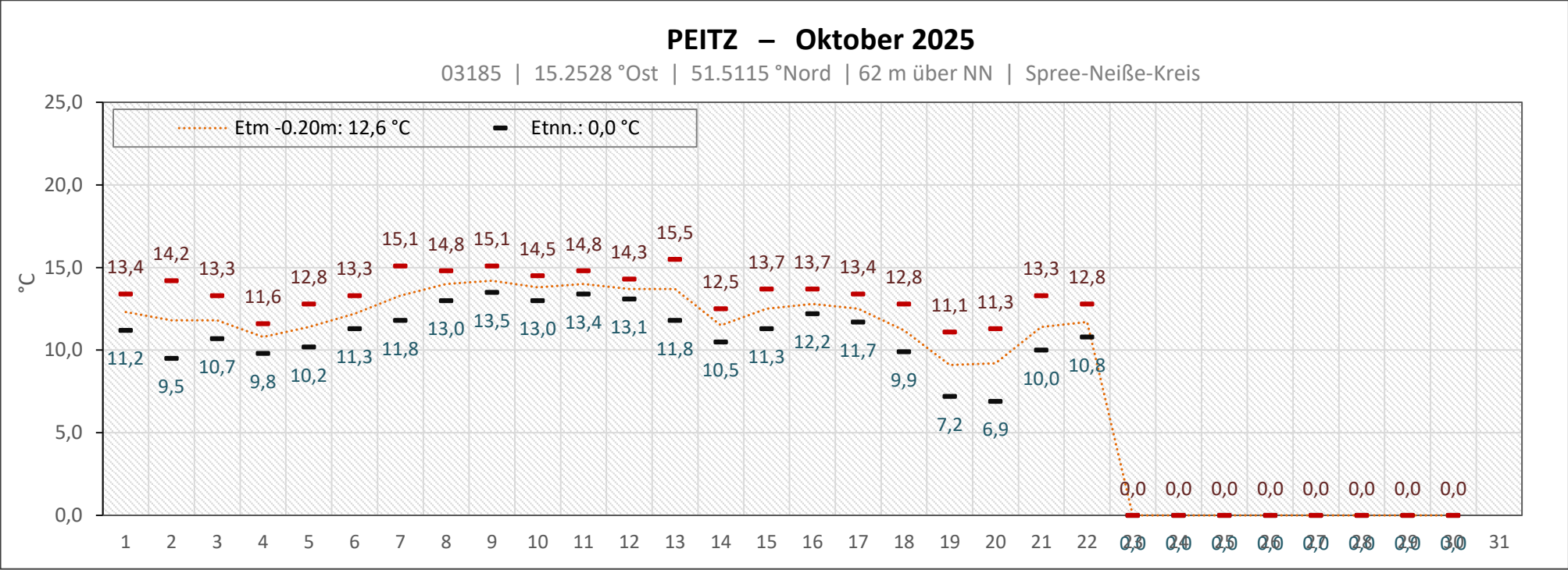
Diagramm der Tageswerte aus 0,20 m tiefe.
