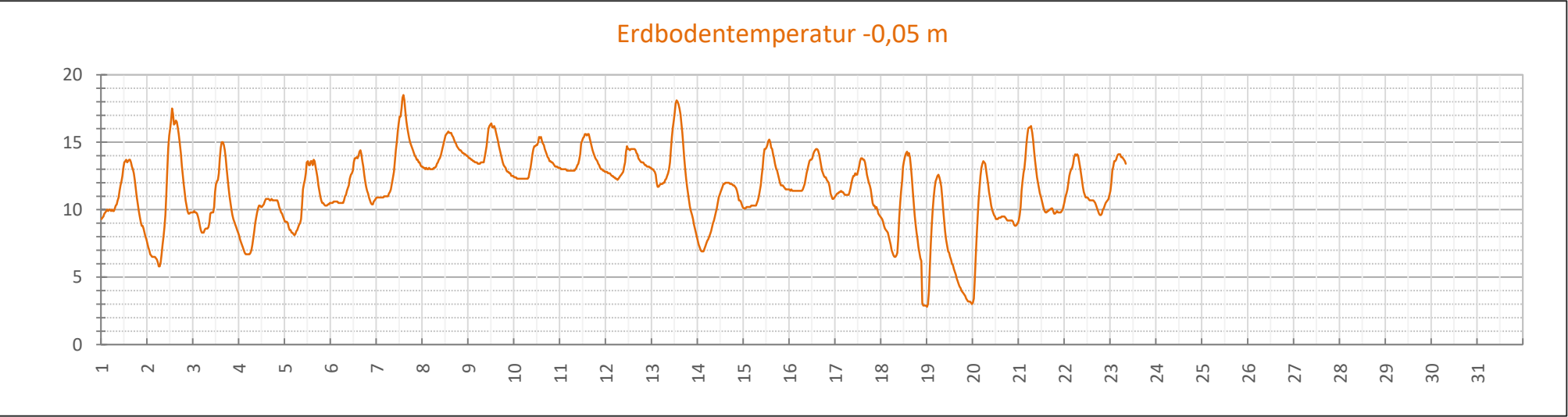
Diagramm der Erdbodentemperatur in 0,05 m tiefe im 10-Min-Takt
