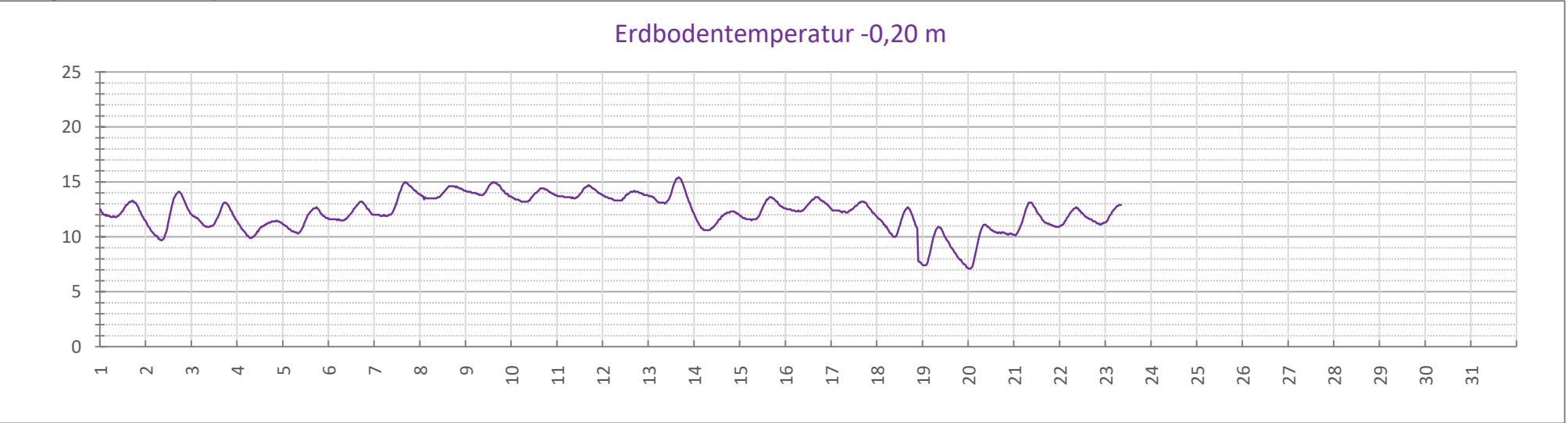
Diagramm der Erdbodentemperatur in 0,20 m tiefe im 10-Min-Takt
