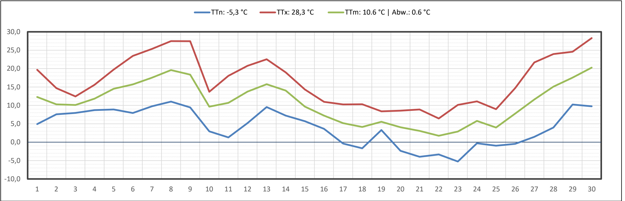
10-Min Temperaturwerte
