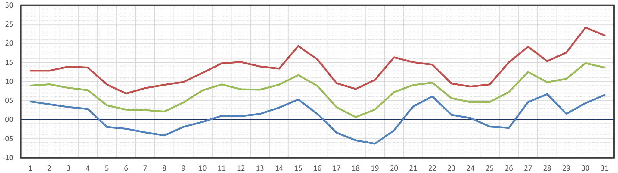
10-Min Temperaturwerte
