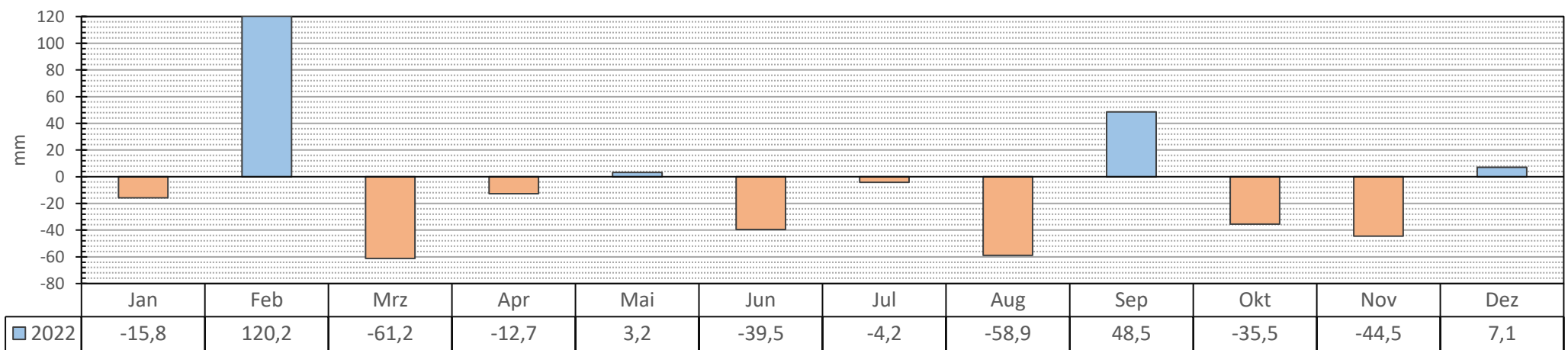
Abweichung Monatsniederschlag 2022 | Hamburg-Horn
